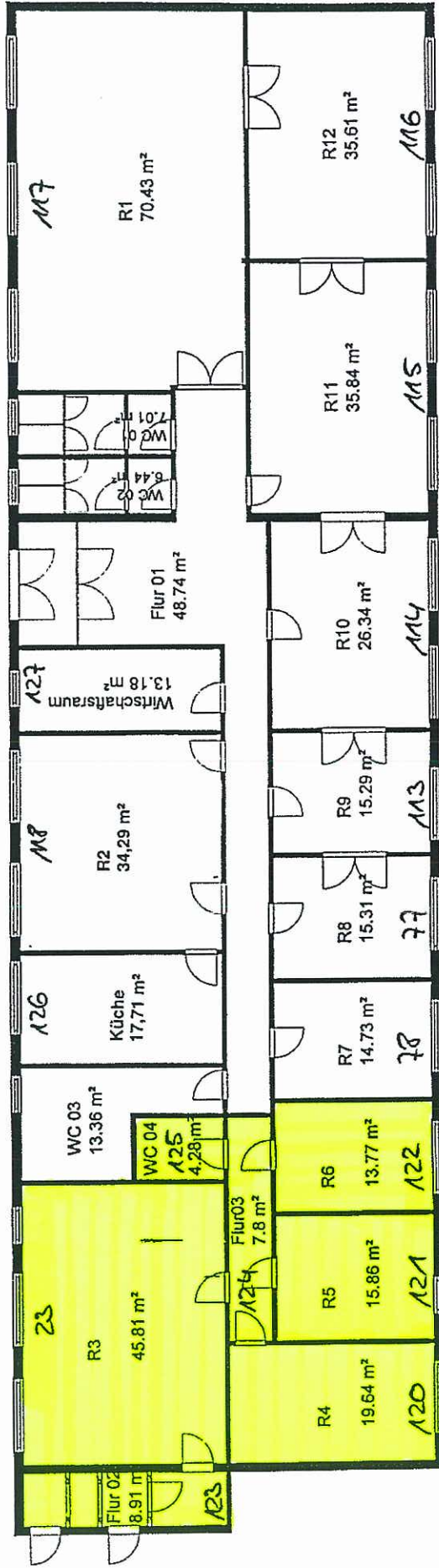
Grundriss Geb. 288 (o. Maßstab)
